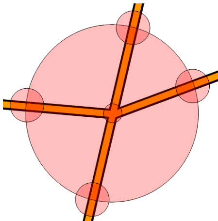
Bild 6: Knotenpunkt mit markierter Konfliktsfläche, Einfluss-, Einfahr- und Ausfahrbereichen zur automatischen Auswertung von GPS-Mitschriften von Fahrzeugflotten
