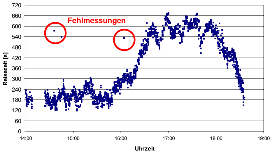
Bild 4: Reisezeiten auf einem Streckenabschnitt (Datenerfassung mittels Kennzeichenerfassungssystemen am Anfang und am Ende der Messstrecke)
